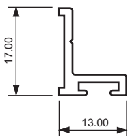
Section No. 6136 Door Stop
