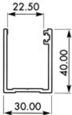
Section No. G673, 0.613 kg/m per 235
