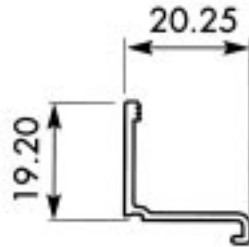
Section No. E771, 0.159 kg/m per 90
