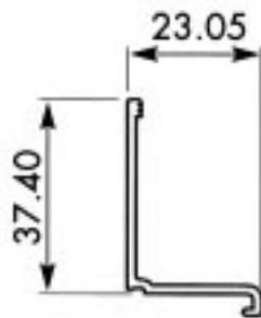
Section No. G674, 0.247 kg/m per 124
