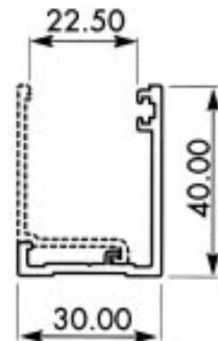
Section No. G675, 0.448 kg/m per 178
