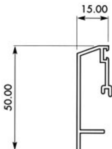
Section No. 30005 0.420 kg/m, per 211.25
