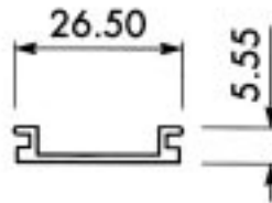
Section No. 8167 Infil 0.139 kg/m, per 85
